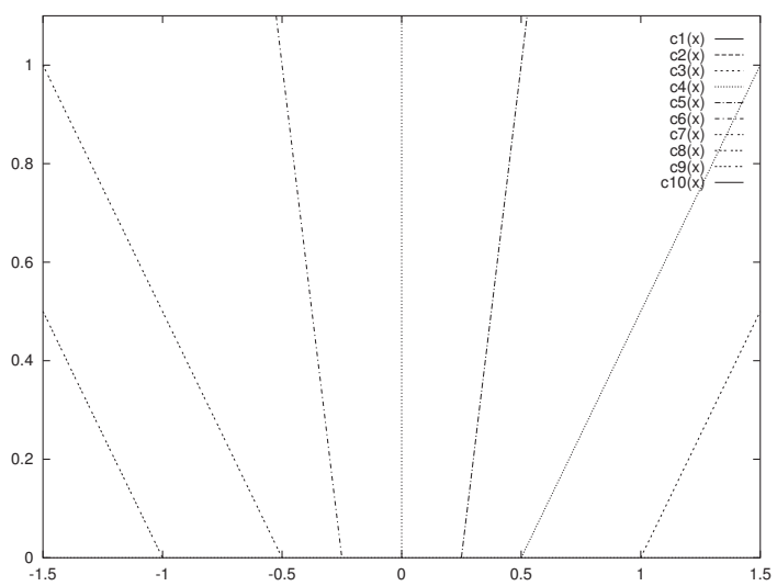
図 7: 青信号後の交通波の特性曲線
