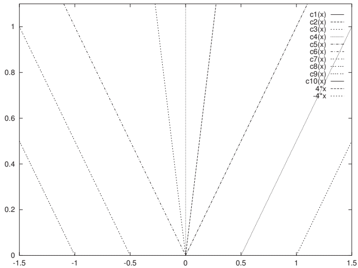
図 9: 青信号直後の希薄波の特性曲線
