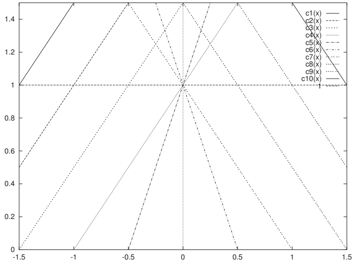
図 5: 赤信号による衝撃波の特性曲線
