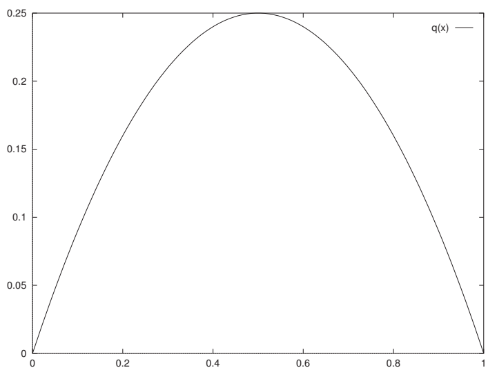
図 2: 線形モデルにおける交通密度・交通流量関係
