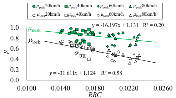
図-4 RRCと \mu_{lock} 、 \mu_{peak}
