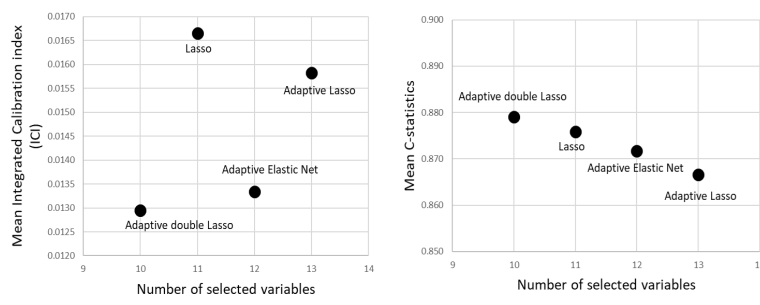
図1 各モデルの性能評価(臨床データ1)
